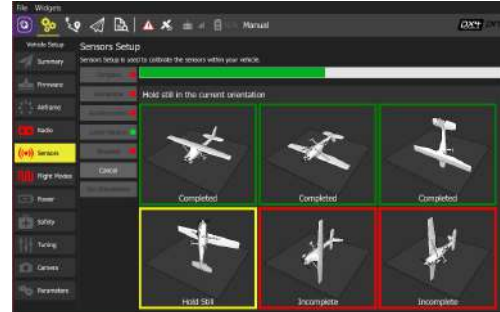
(b) Calibración del acelerómetro en QGroundControl .
