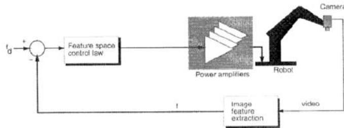
Figura 3.52: Sistema de Visual Servoing basado en imágenes.
