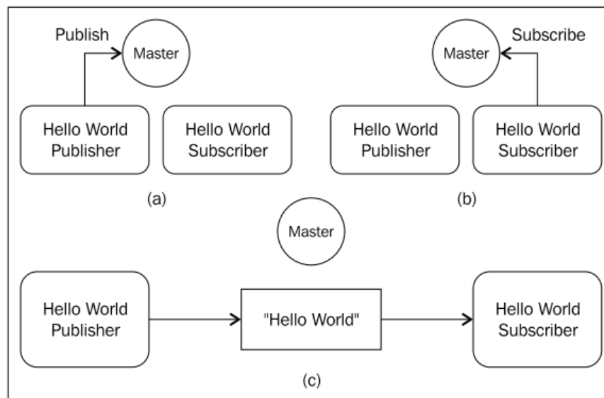
Figura 3.47: Interacción del ROS Master.
