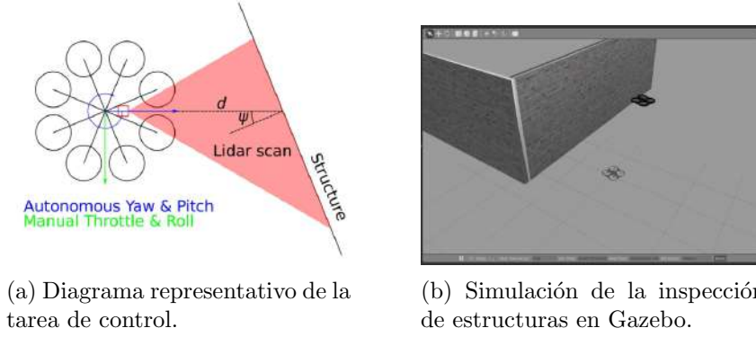
Figura 2.5: Inspección de estructuras utilizando drones con ROS y Gazebo.
