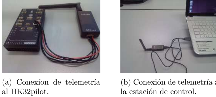
Figura 3.29: Sistema de telemetría.
