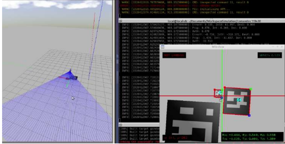
Figura 5.13: Vista de simulación para la detección de marcadores de Aruco.
