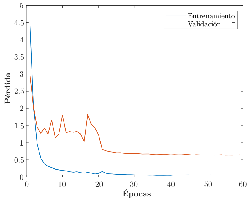
Figura 3.3: Gráfica de la función de pérdida durante el entrenamiento de la EfficientNet-B0 en los conjuntos de entrenamiento y validación.
