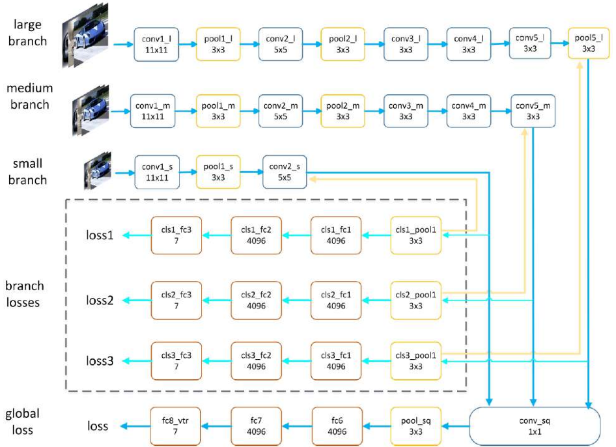
Figura 1.3: Modelo CNN con retroalimentación de múltiples ramas basado en AlexNet propuesto por Chen et al. tomado de [2].
