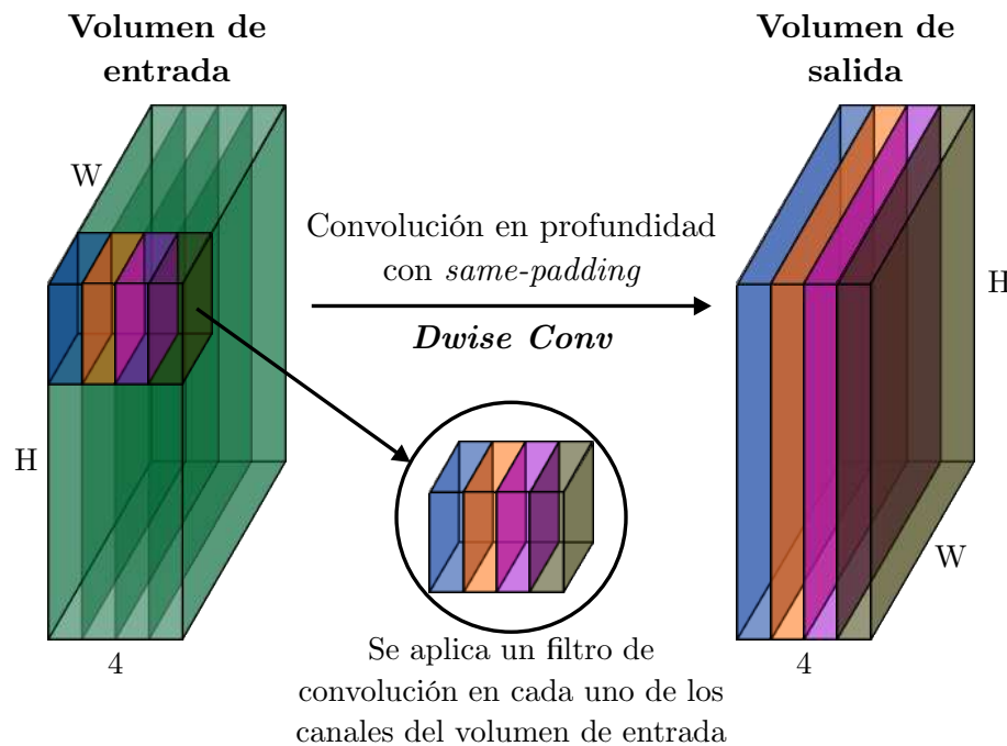
Figura 2.15: Convolución en profundidad con same-padding sobre un volumen de H \times W \times 4 .
