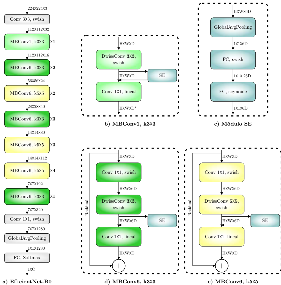
Figura 2.16: Arquitectura de la EfficientNet-B0 [3]. En a) se observa el diagrama general de la arquitectura completa. En b), d) y e) sus respectivos cuellos de botella invertidos móviles MB-Conv [4]. Y en c) el módulo SE ( squeeze-and-excitation ) [5].
