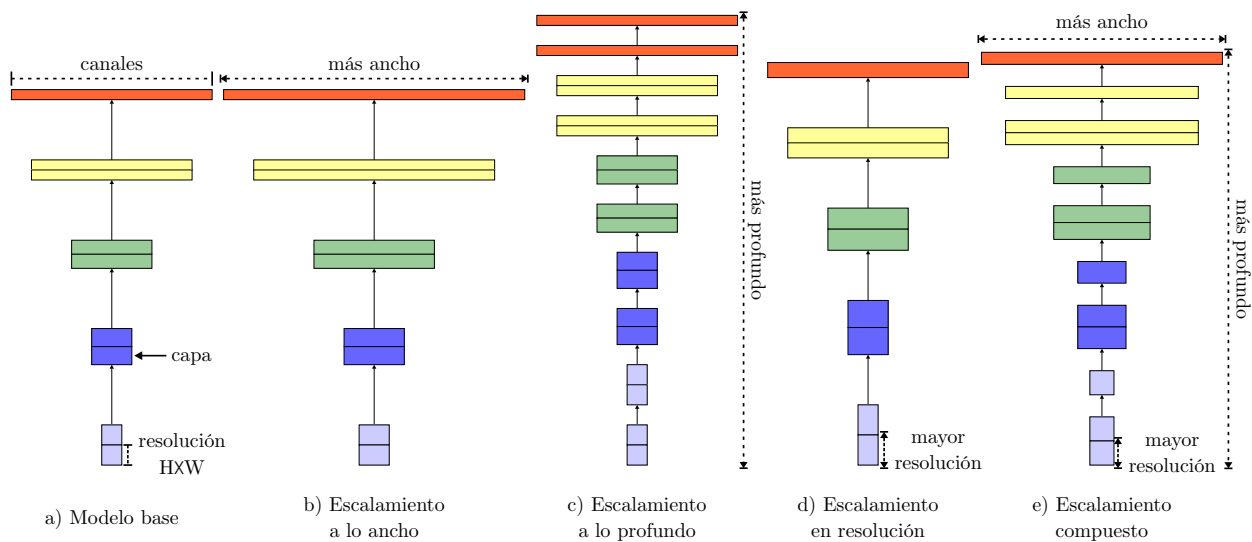
Figura 2.14: Diferentes tipos de escalamiento de CNN. a) Es el modelo base de CNN, b)-d) son escalamientos convencionales y, e) es el escalamiento propuesto por Tan y Le [3].
