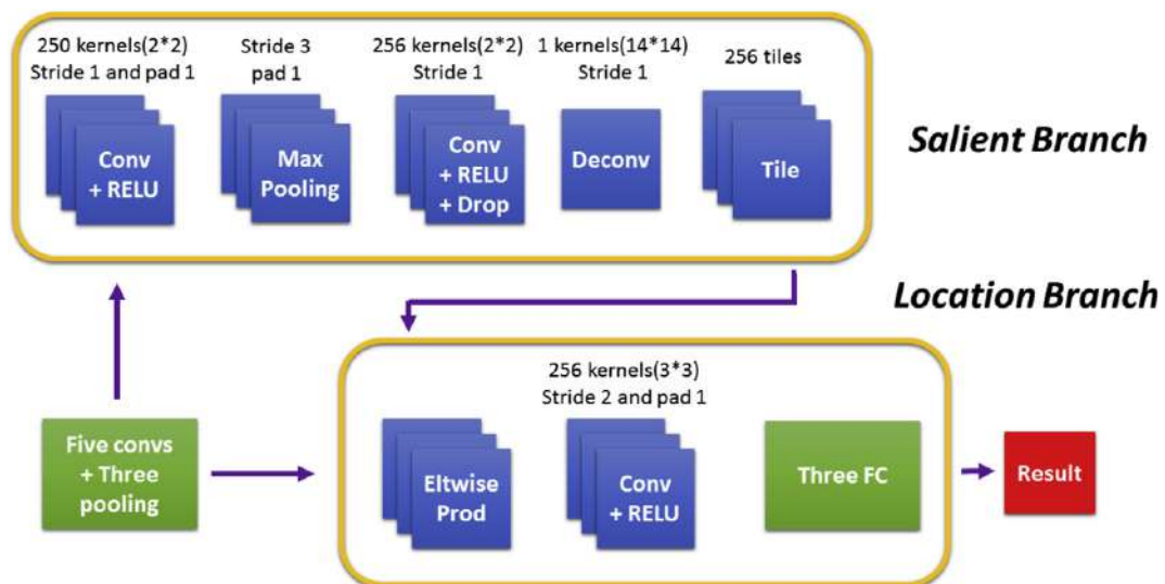
Figura 1.1: Arquitectura de la red de localización de Hu et al. tomado de [1].
