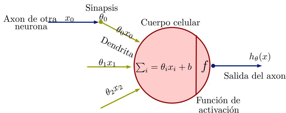
Figura 2.2: Modelo matemático de una neurona.
