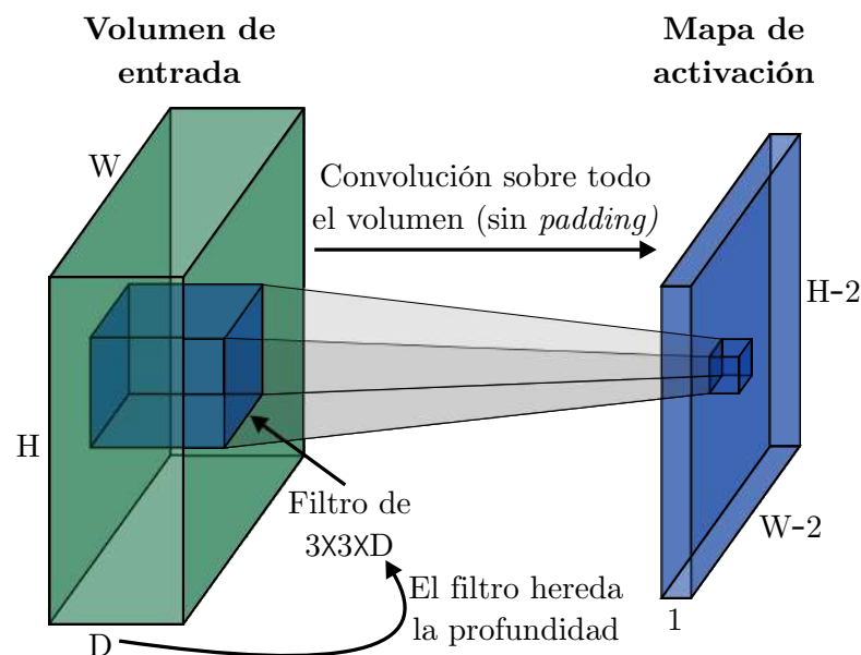
Figura 2.11: Obtención de un mapa de activación con un filtro de convolución de 3 \times 3 sobre un volumen de entrada H \times W \times D , sin aplicar padding .
