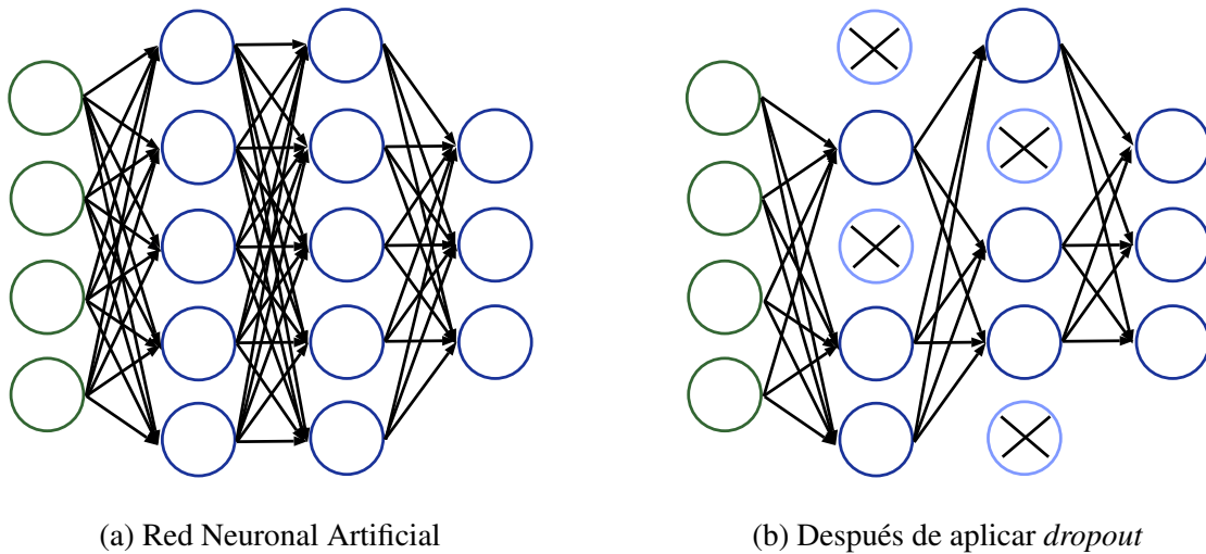
Figura 2.7: Ejemplo de red neuronal artificial y el resultado de aplicarle dropout .
