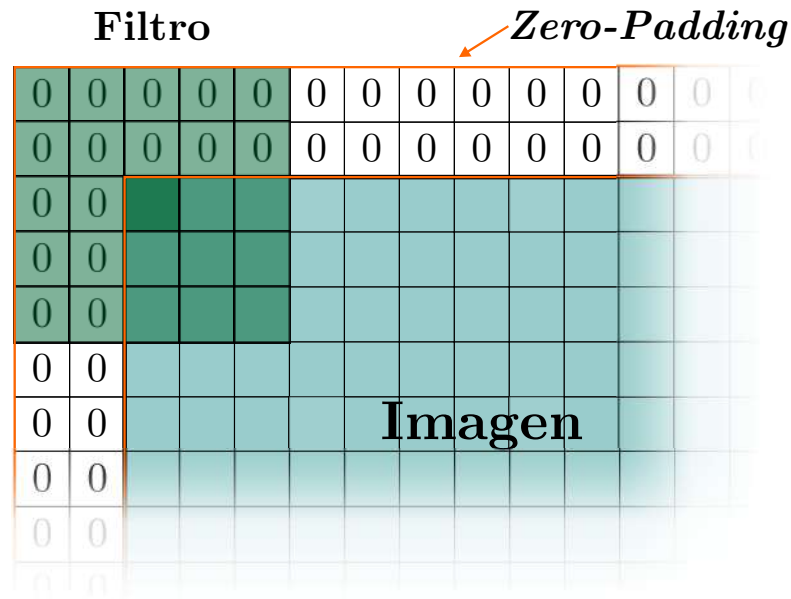
Figura 2.10: Zero-padding sobre una imagen a la que se le aplica un filtro de convolución de 5 \times 5 .
