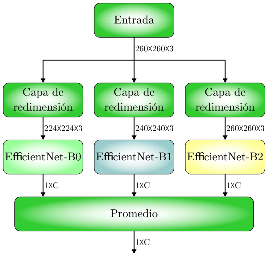
Figura 3.1: Modelo propuesto, Ensemble de EfficientNets.
