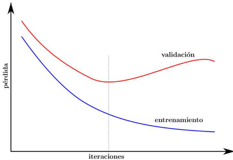
Figura 2.6: Curvas de la función de pérdida con overfitting .
