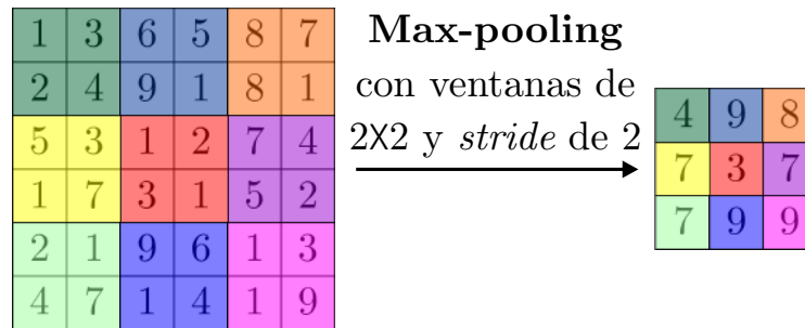
Figura 2.13: Max-pooling sobre un arreglo de 6 \times 6 con ventanas de 2 \times 2 y stride de 2, que da como resultado un arreglo de 3 \times 3 .
