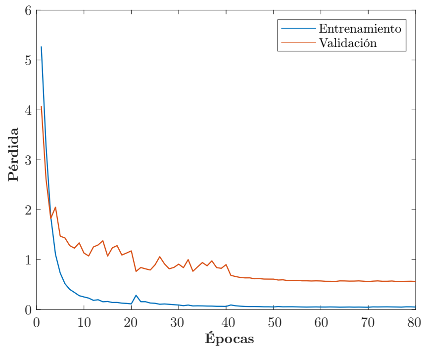
Figura 3.5: Gráfica de la función de pérdida durante el entrenamiento de la EfficientNet-B2 en los conjuntos de entrenamiento y validación.
