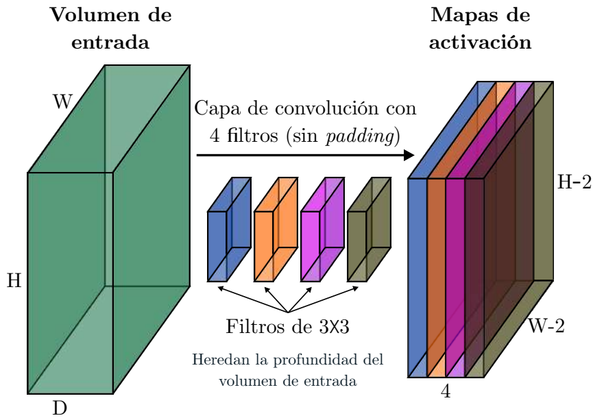
Figura 2.12: Obtención de mapas de activación con una capa de convolución de 4 filtros de 3 \times 3 sobre un volumen de entrada H \times W \times D , sin aplicar padding .
