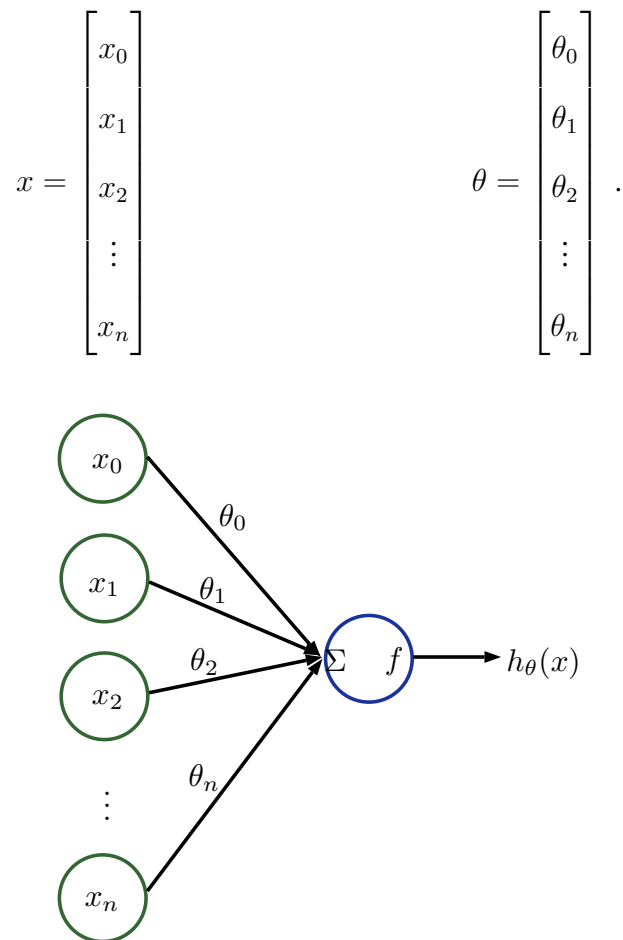
Figura 2.3: Representación de una neurona artificial.
