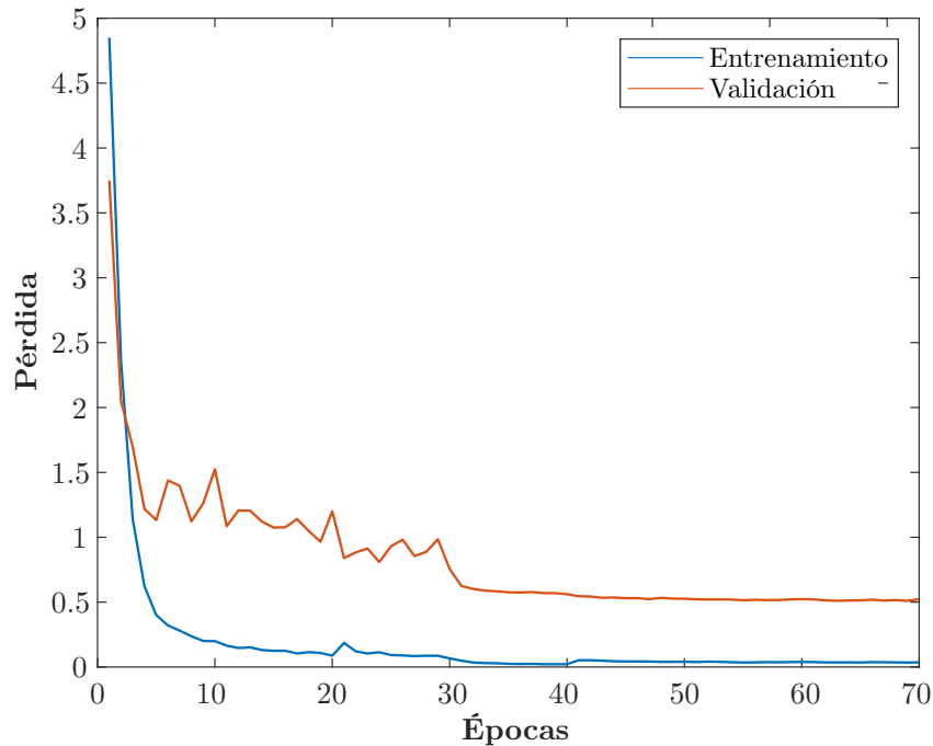
Figura 3.4: Gráfica de la función de pérdida durante el entrenamiento de la EfficientNet-B1 en los conjuntos de entrenamiento y validación.
