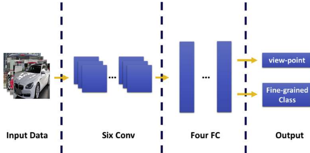
Figura 1.2: Arquitectura de la red de reconocimiento de Hu et al. tomado de [1].
