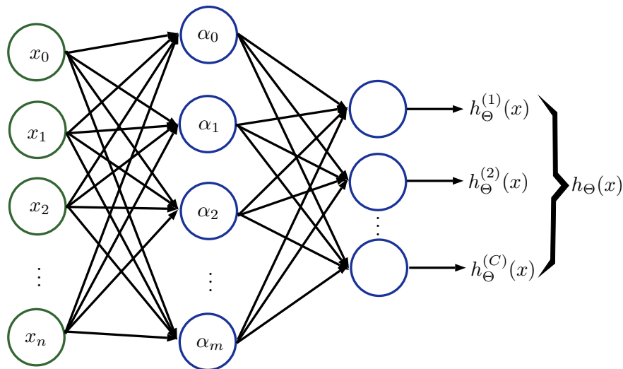
Figura 2.5: Representación de una red neuronal artificial multiclase.
